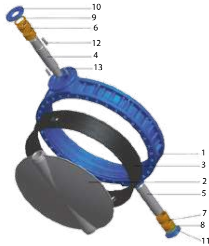
DN1400-1800
