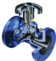
Βαλβίδα Τύπου A Valve Type A
