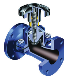
Βαλβίδα Τύπου KB Valve Type KB
